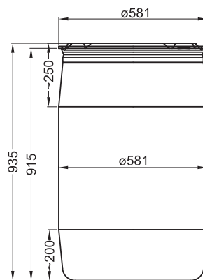
Standaard plasticen vat (DS/EN 12707).
