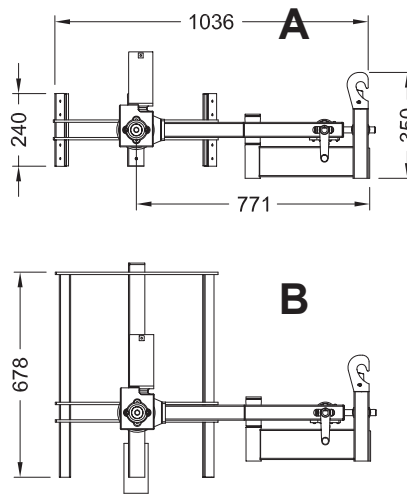
B: Vatenkantelaar voor standaard plasticen vaten (DS/EN 12707).
